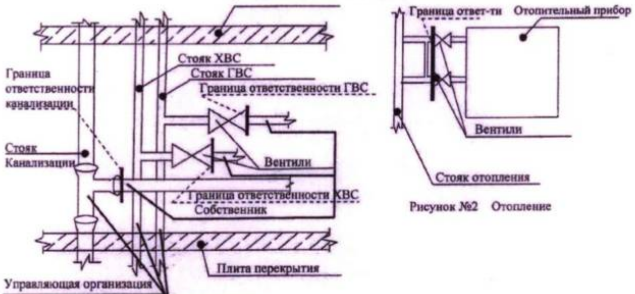
Рисунок № 1. Водоснабжение и канализация.
